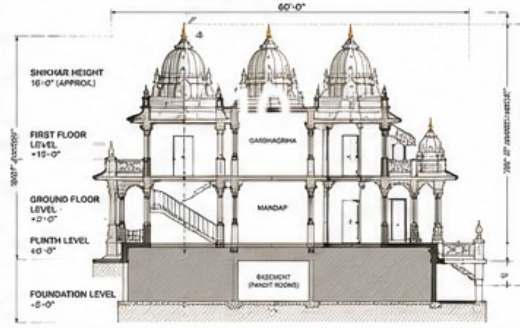
10. SECTION (A-A)
